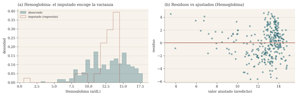
Figura 4: Imputación de los datos
